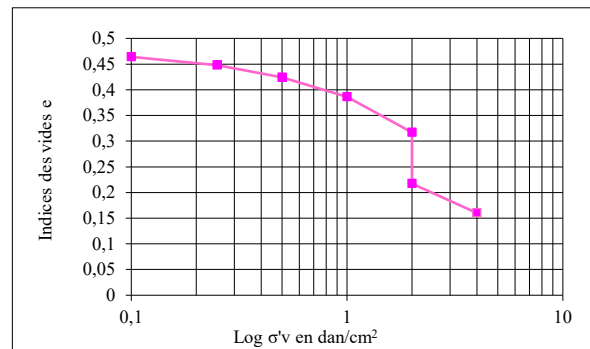
Figure. 2. Courbe de compressibilité du sol testé selon la procédure Knight (1975)
