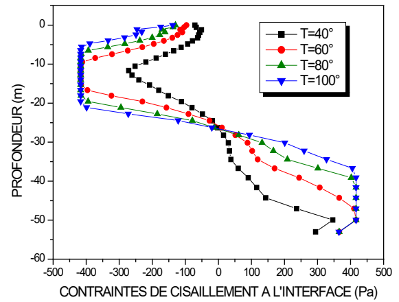
Figure.8. Évolution des contrainte de cisaillement à l'interface en fonction de la variation de la température.
