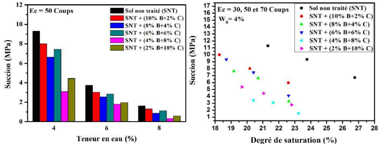
Figure. 1. Effet du mélange bentonite-ciment sur la pression capillaire
