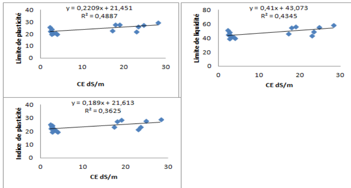
Figure 2. relation entre la CE et les de liquidité de plasticité et l'indice de plasticité
