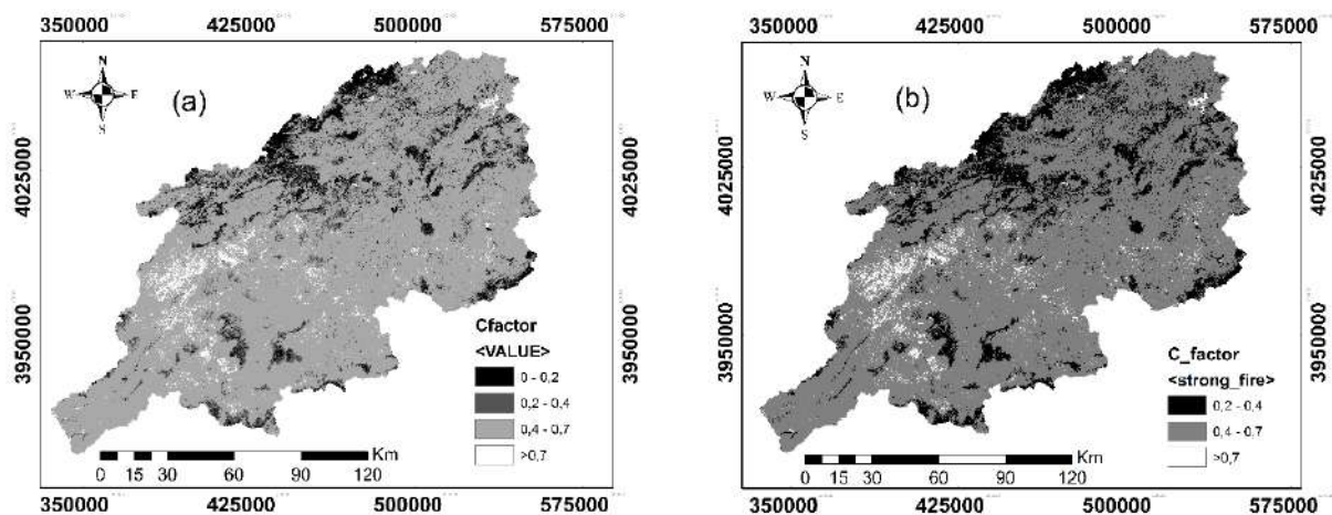
Figure 3. Le facteur C du modèle RUSLE selon les deux scenarios (a/actuel. b/incendie)
