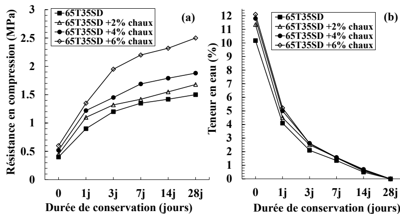
Figure.2. Evolution de : la résistance à la compression (a) et de la teneur en eau (b) en fonction de la durée de conservation.
