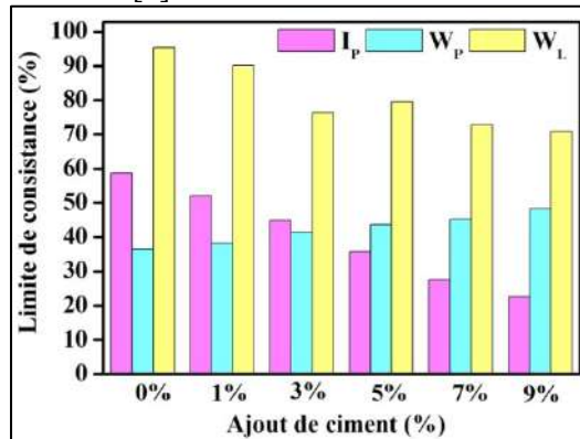
Figure. 1. Résultat des limites de consistance de sol avant et après traitement.
